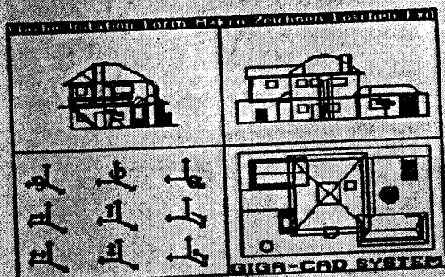
Obr. 9 Dům pro konstrukci ve vstupní jednotce.
